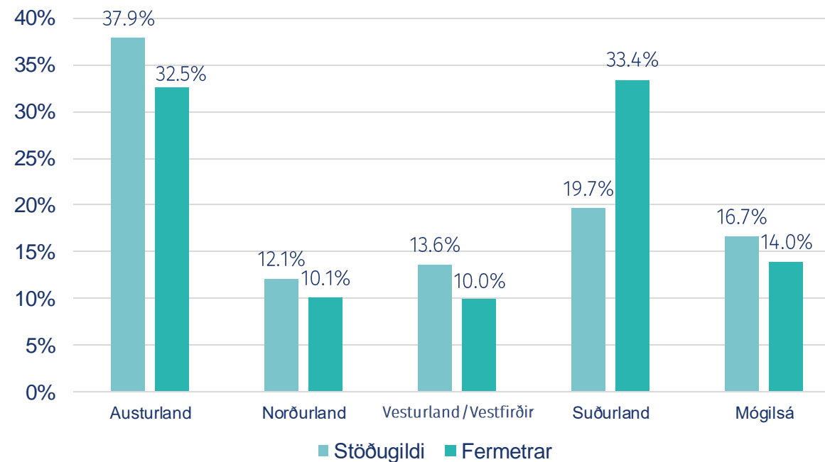
Starfsstöðvar Skógræktarinnar
